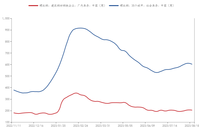
图 1. 螺纹钢社库、厂库均小幅回落（万吨）
