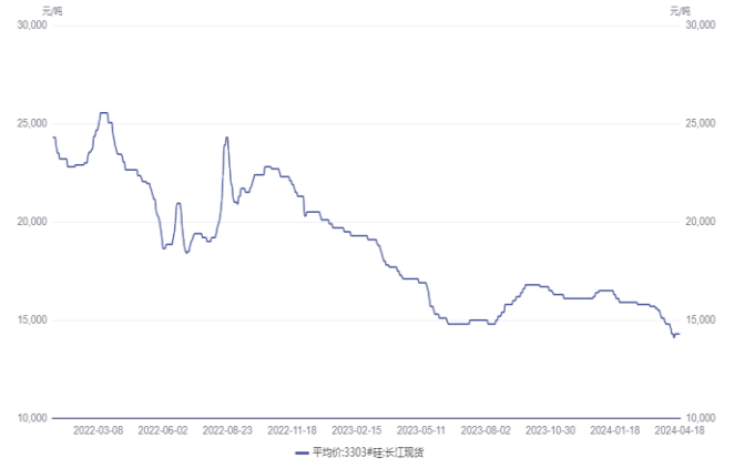
图 2. 工业硅 3303#价格走势（元/吨）
