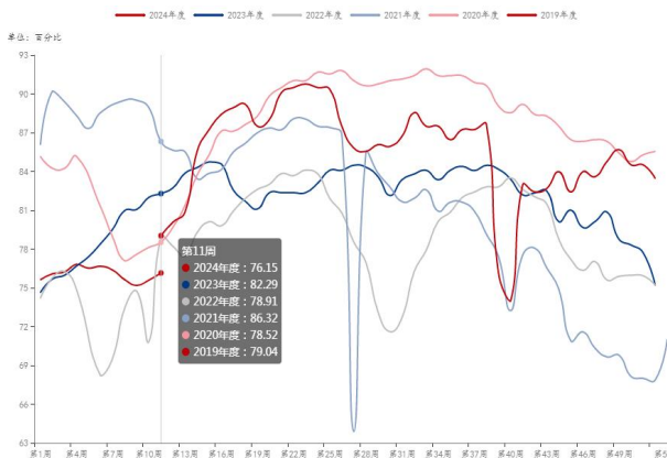
图 4. 高炉开工率处于近年低位 (%)
